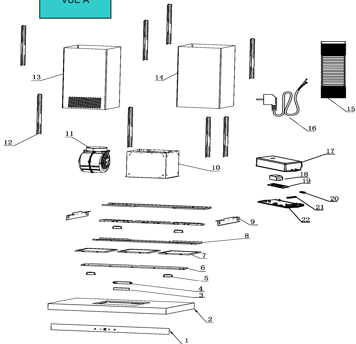
VUE A
