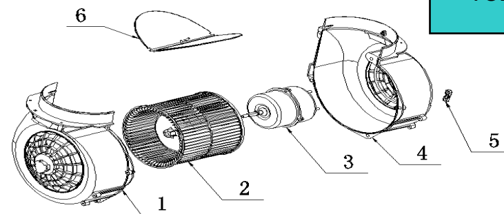
VUE B
